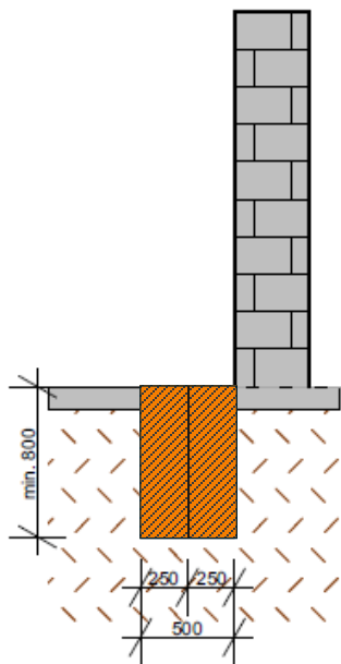
Bočný pohľad
