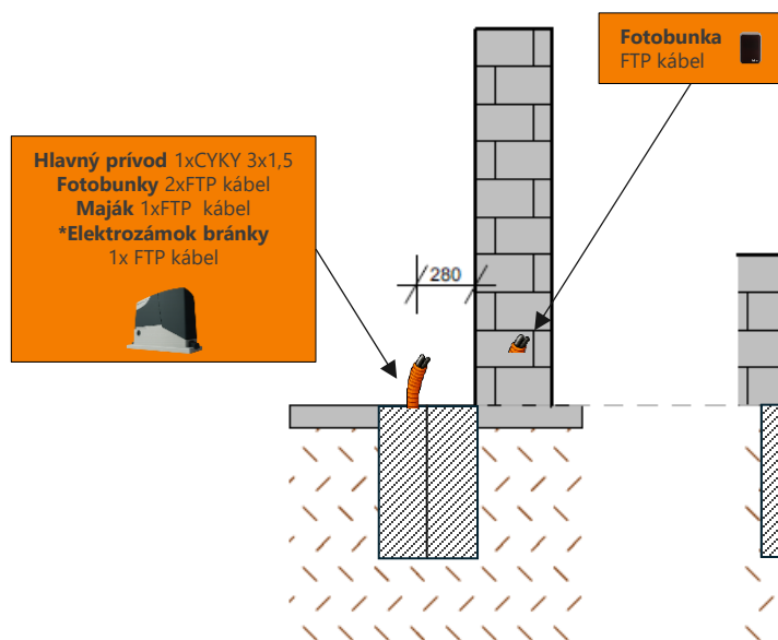
Bočný pohľad
